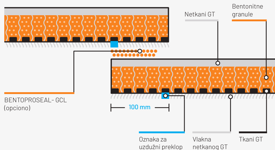
Slika 1. / BENTOCARPET V5, šematski prikaz proizvoda na uzdužnom preklapu
