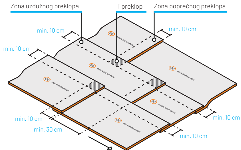
Slika 6. / BENTOCARPET V5, prikaz preklapanja
