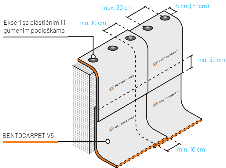
Slika 5. / BENTOCARPET V5, uzdužni preklop na vertikalnom zidu
